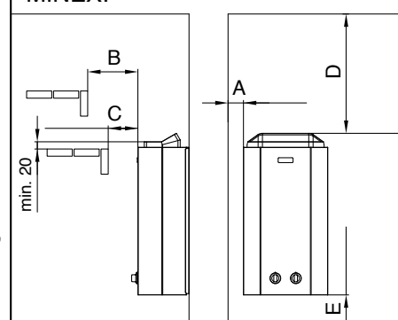
Kuva 1. Kiukaan suojaetäisyydet
