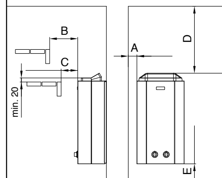
Рисунок 1. Безопасные расстояния для каменки.
